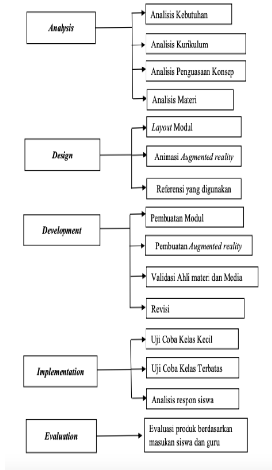
Gambar 1 Desain Penelitian
